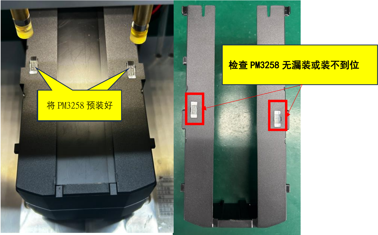
图二，将 PM3086 先放入治具，在将两个 PM3258 预装好，再进行压合， 压合到位后取出检查物料无漏装或压合不到位。
