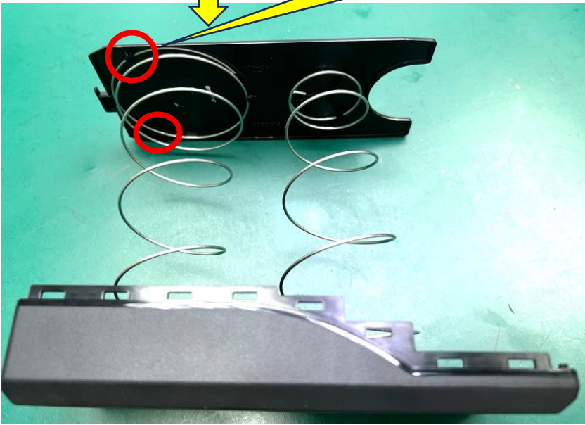
图一，将 PA3577-3 和 PA3577-4 装配在一起，注意装配方向，将弹簧大口位装入卡扣，确保弹簧开口处 2 个扣完全扣入。
